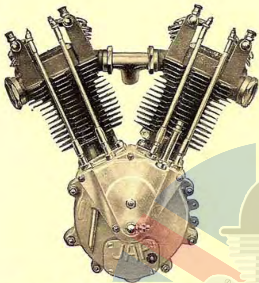
750 c/c. Culbuteurs "RACING"
